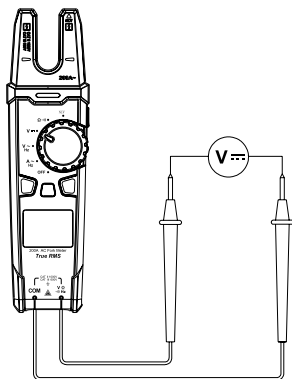
Рис 4. Измерение напряжения постоянного тока
