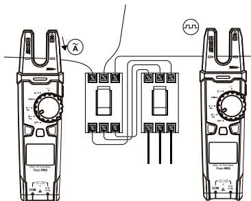
Рис. 3 Измерение переменного тока и частоты
