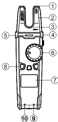
Рис.1 Общее устройство
